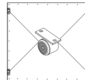
Рис.3 Монтаж колесных опор Выдвижной ящик. Вид снизу
