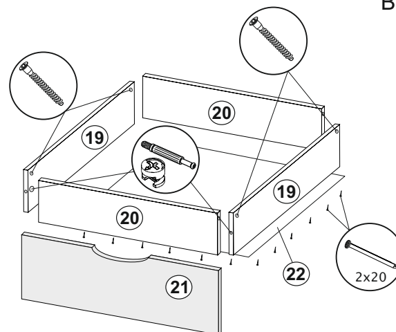
Рис.2 Сборка выдвижного ящика
