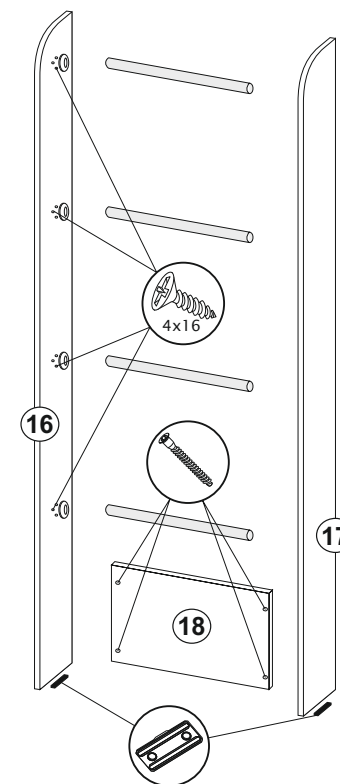
Рис.4 Сборка лестницы
